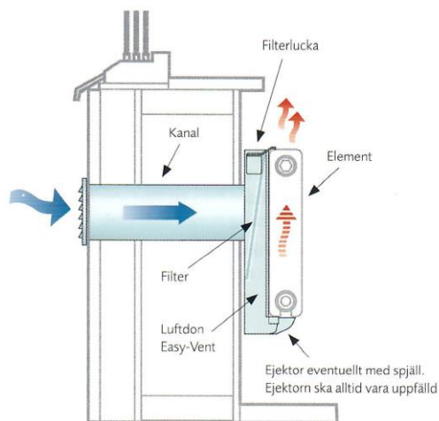
Vägg i genomskärning med kanal och luftdon Easy-Vent med monterat element (radiator)
